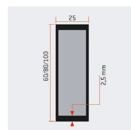
Perfiles de sección reforzada 2,5 mm.
