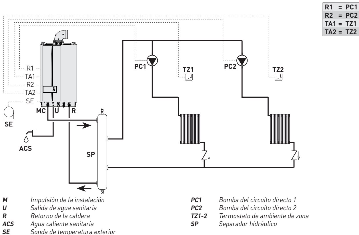
Tipo 1: Instalación con dos circuitos directos multizona
