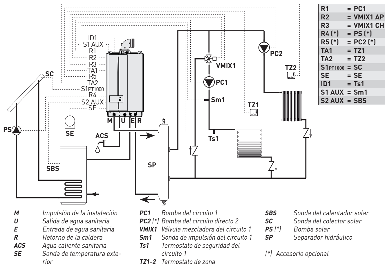
Tipo 10: Instalación con caldera instantánea con un circuito directo multizona, un circuito mezclado multizona y calentador solar remoto para precalentamiento de agua sanitaria
