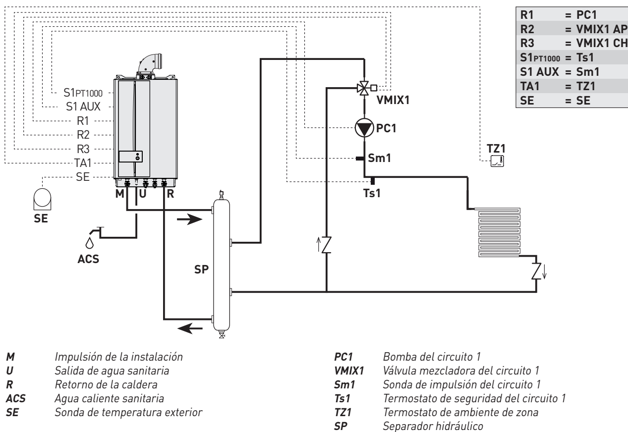
Tipo 2: Instalación con un circuito mezclado multizona
